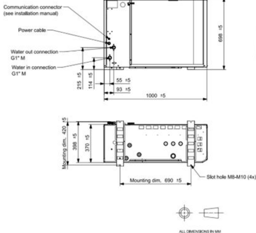
Aansluitingen van de Flint
