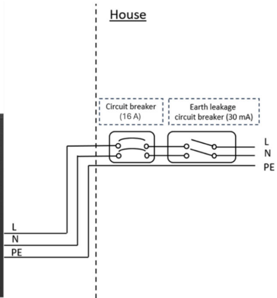
Stroomvoorziening elektrisch schema - Flint
