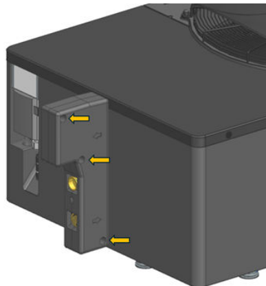
Montage van de appendage isolatie
