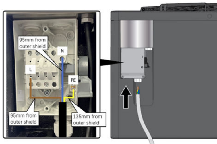
Stroomvoorziening aansluiten (230V - 16A)
