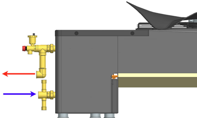
Aansluiting van de aan- en afvoer in de Blackbird
