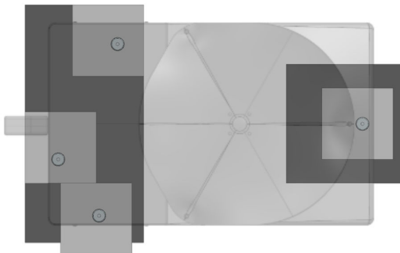
Tegelloccatie (bovenaanzicht) - 4x tegels van 30x30cm (grijs) of 3x tegels van 50x50cm (zwart)
