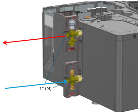
Aansluiting van de aan- en afvoer in de Blackbird
