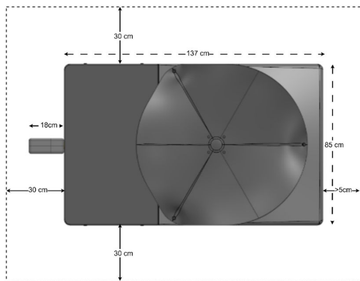
Vrije ruimte rondom de Blackbird
